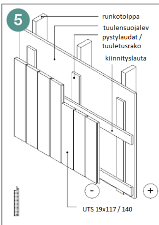
5 Příklad vertikálního obkladu.
