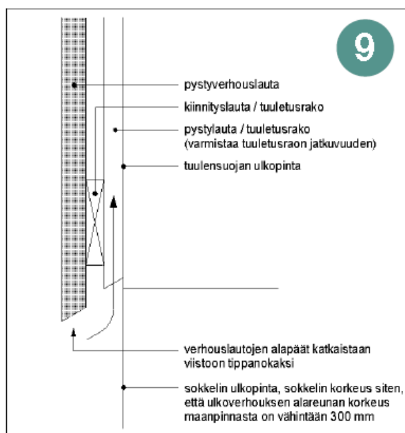
9 Spodní okraj vertikálního obložení / větrací štěrbina. Spodní konce palubek se zkrátí zešikma, aby vznikl odkapávací profil, a pečlivě se ošetří nátěrem.
