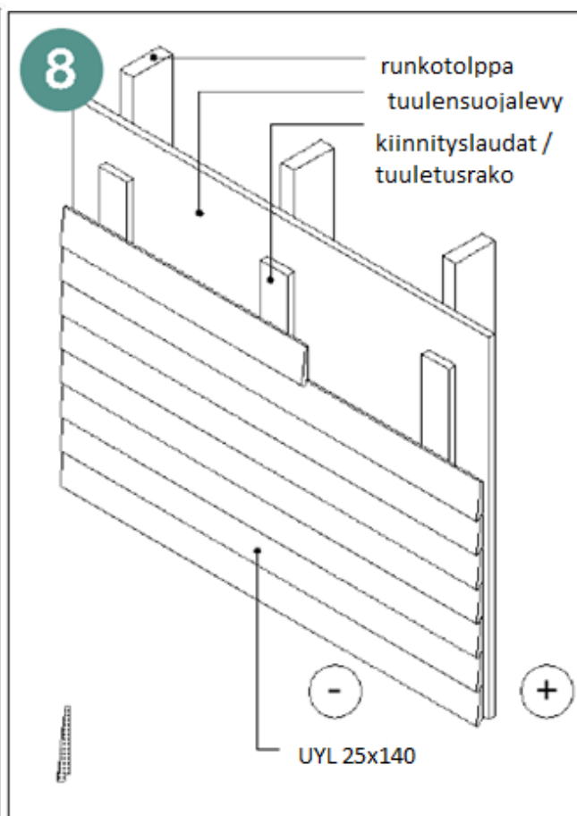
8 Příklad horizontálního obkladu z palubek s překrytím.
